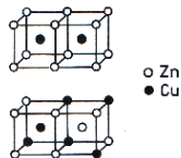
Phasenübergang in \beta -Messing
